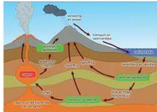
Schematische weergave van de gesteentekringloop
